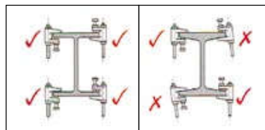
Cách lắp đặt KẸP XÀ GỒ PTTG
