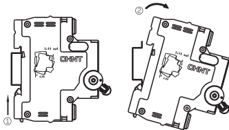
TH35-7.5 DIN Rail
