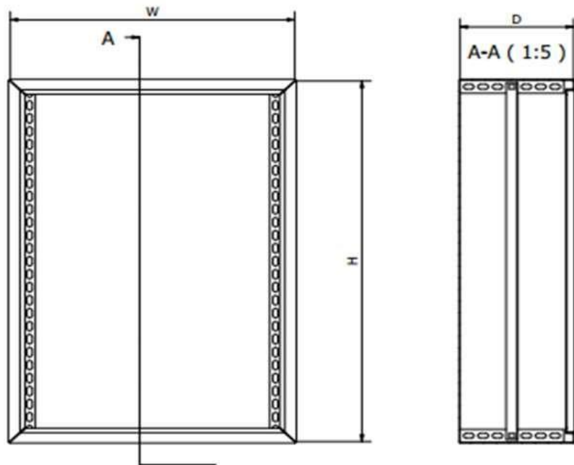
BẢN VẼ TỦ ĐIỆN MD TRONG NHÀ DÙNG THANH CÀI
