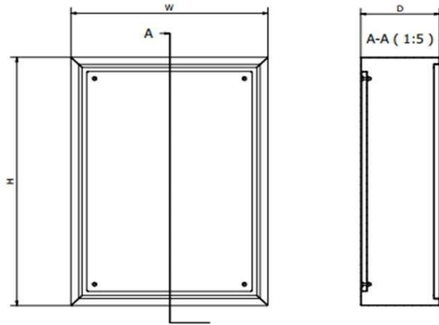
BẢN VẼ TỦ ĐIỆN MD TRONG NHÀ DÙNG TẤM PANEL
