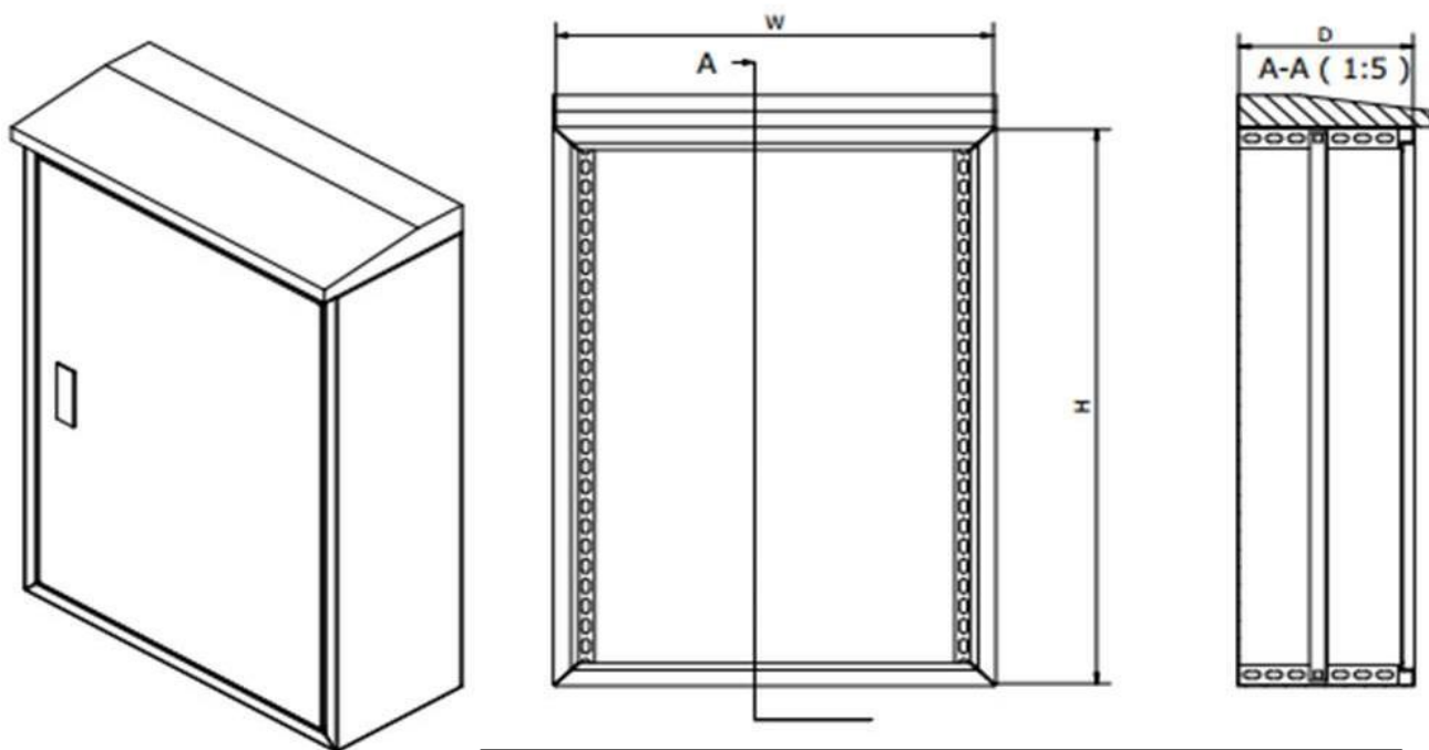
BẢN VẼ TỦ ĐIỆN MD NGOÀI TRỜI DÙNG THANH CÀI
