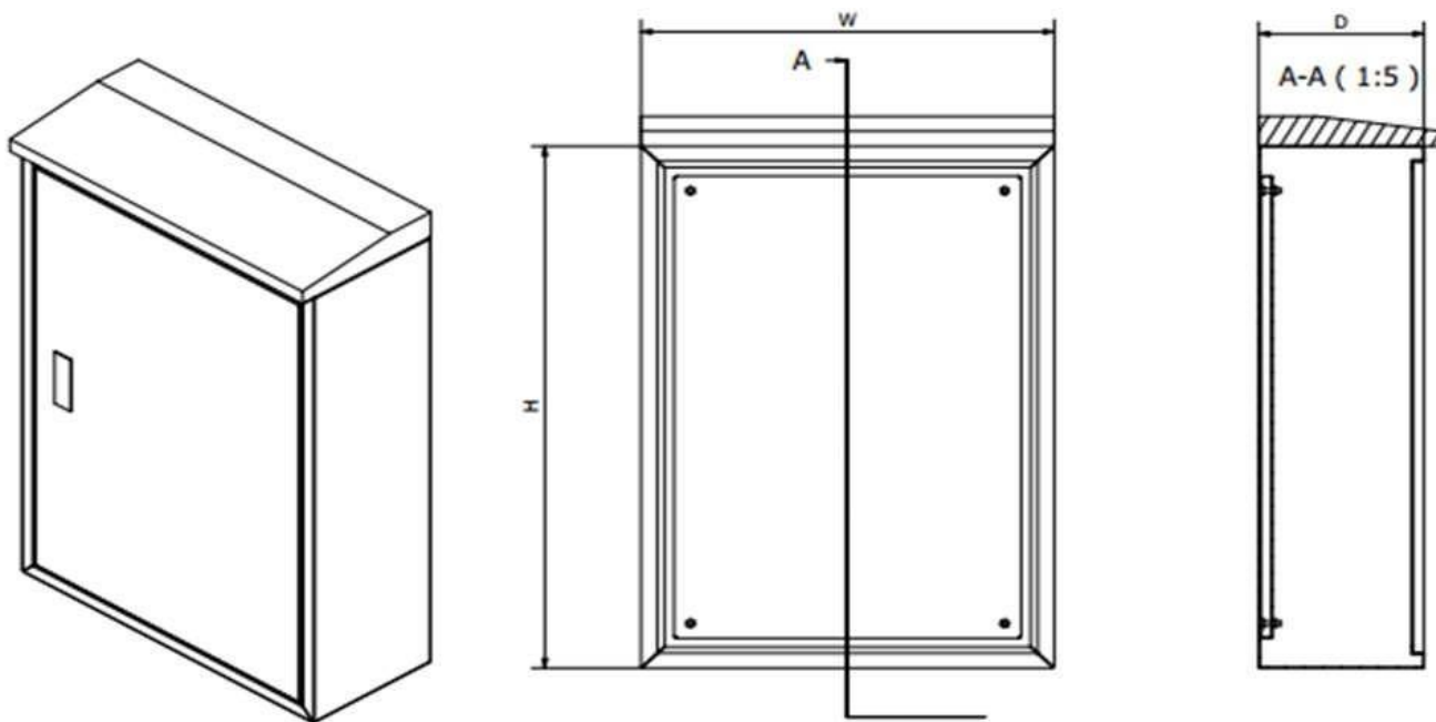
BẢN VẼ TỦ ĐIỆN MD NGOÀI TRỜI DÙNG TẤM PANEL
